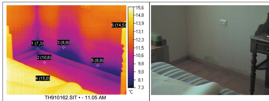
INDAGINE TERMOGRAFICA PER RILIEVO UMIDITÀ
